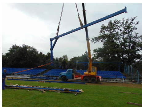
Budowa zadaszenia trybun na Stadionie Miejskim w Skoczowie
